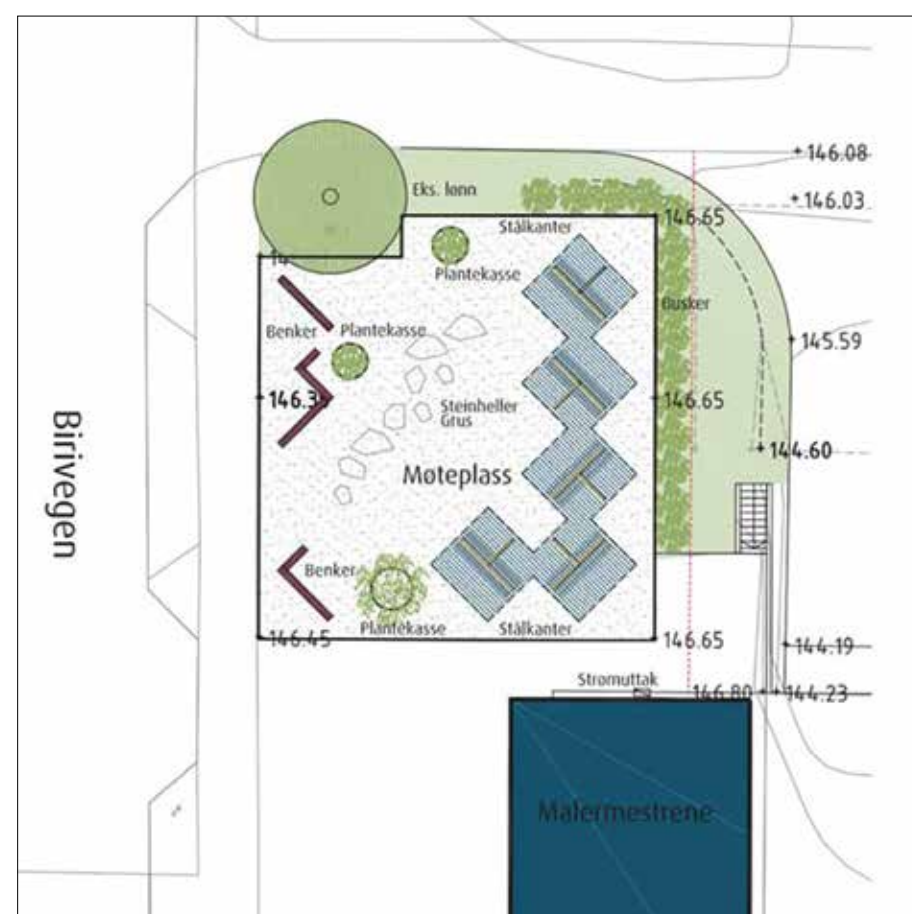
MIDLERTIDIG: Sånn har RAM Arkitektur tenkt at den midlertidige møteplassen i Biri skal se ut. Firkantene på høykant er sitteplasser med glasstak.
